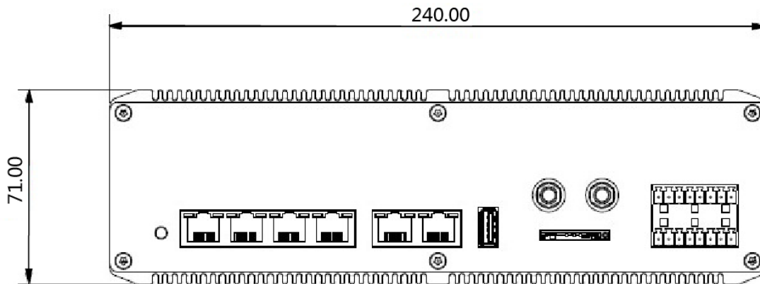
图1-2 侧面板尺寸图（单位：mm）
