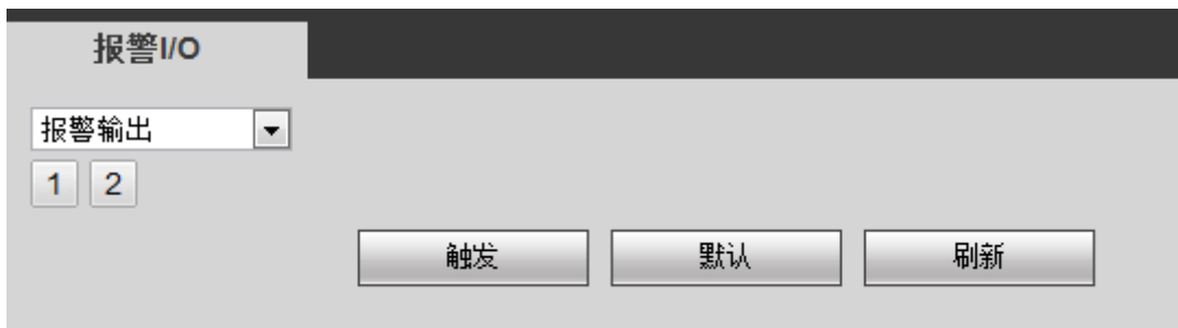
图3-46 报警 I/O
