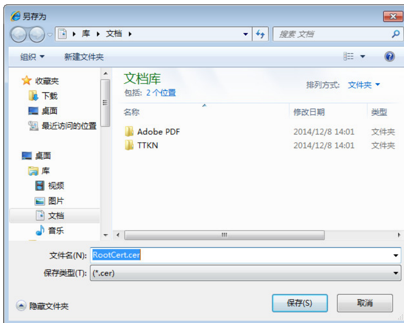
图3-27 下载根证书
