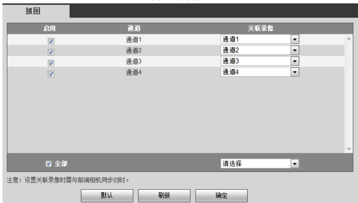
图3-53 抓图设置
