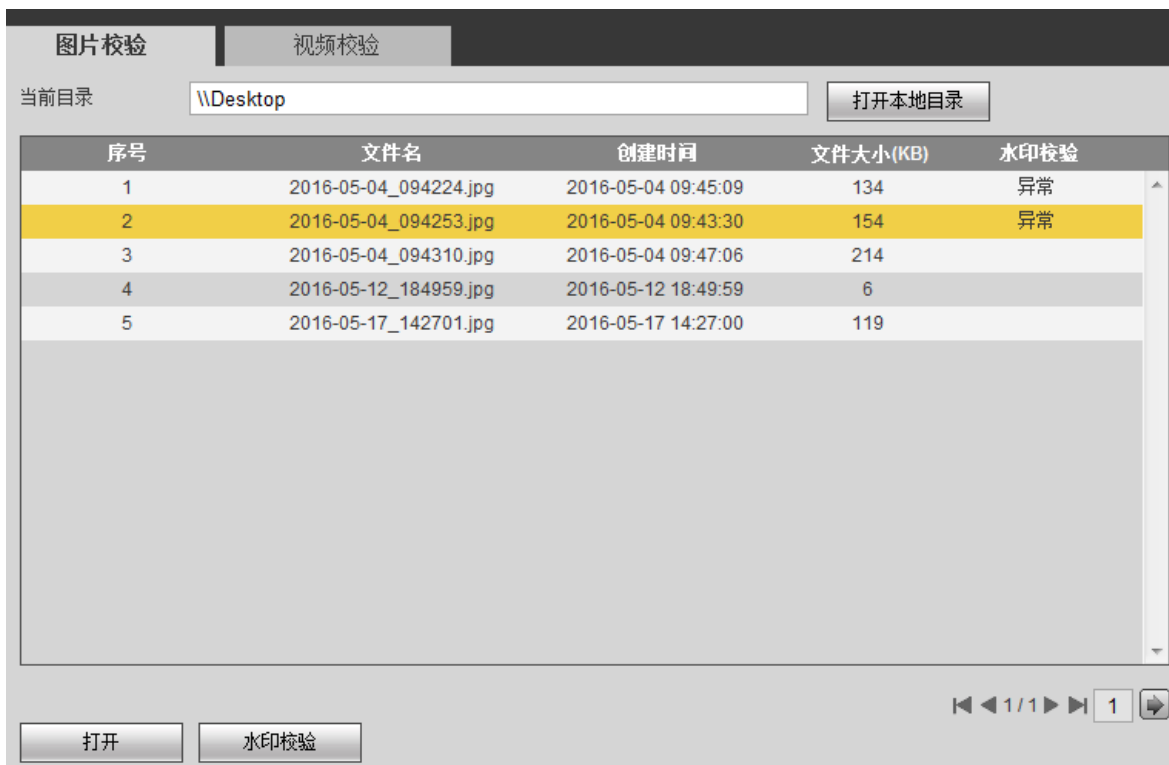
图3-18 图片校验
