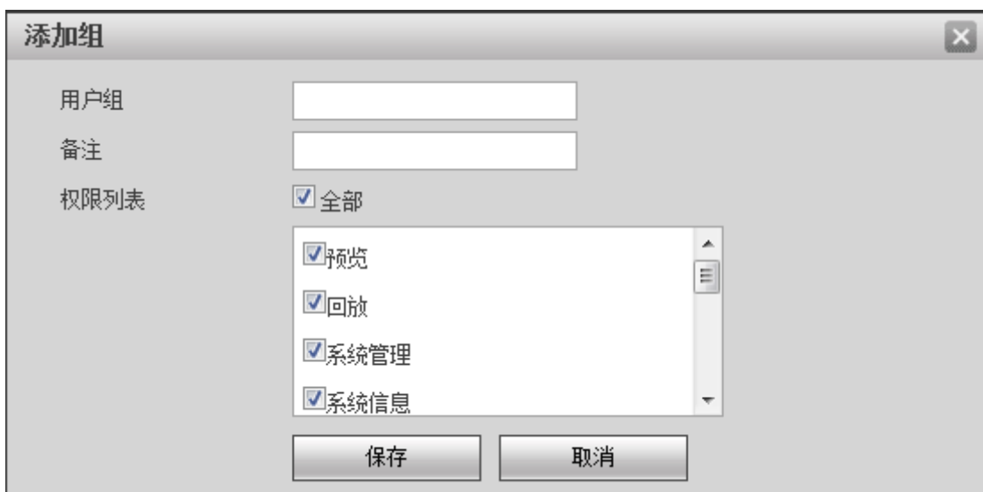
图3-60 添加组
