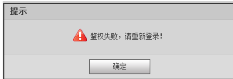
图2-15 提示
