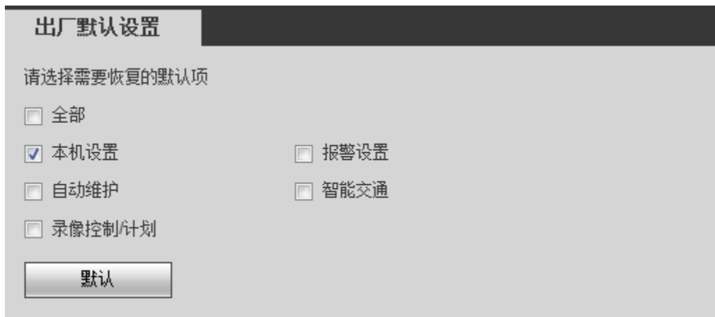
图3-67 默认
