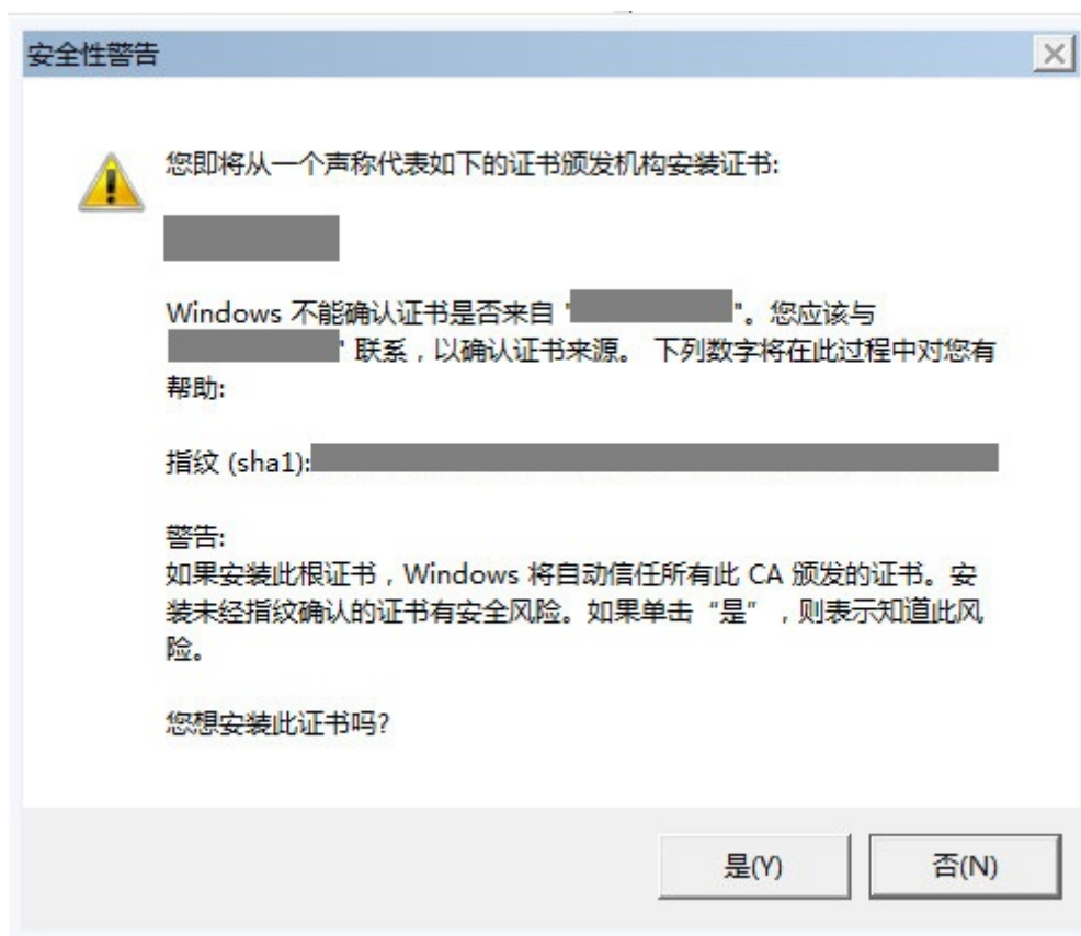
图3-32 安全性警告
