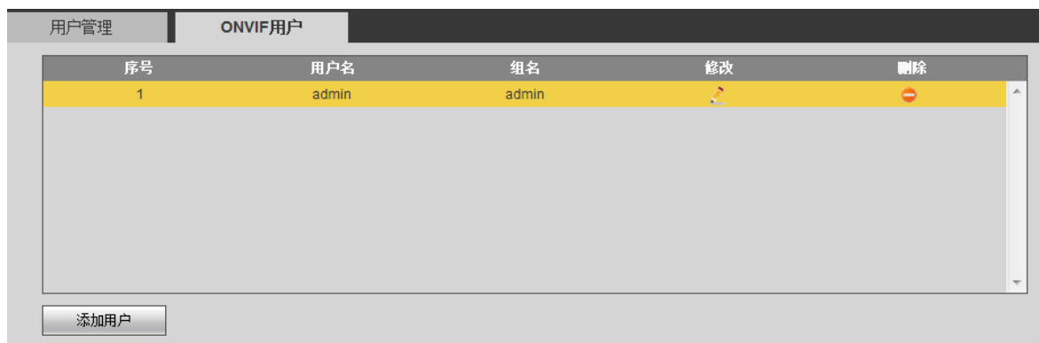
图3-61 ONVIF 用户
