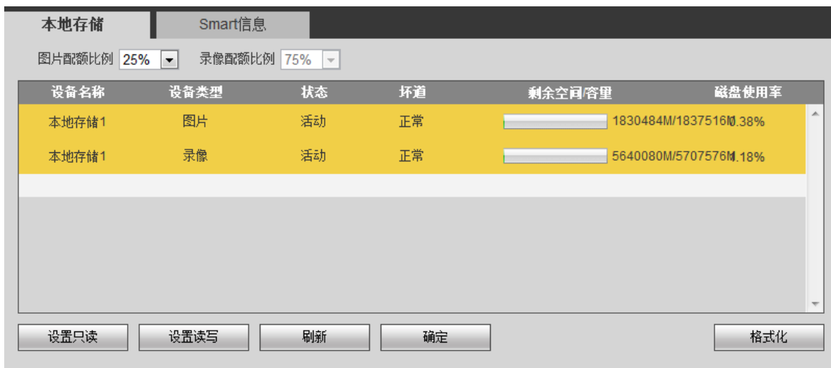
图3-47 本地存储
