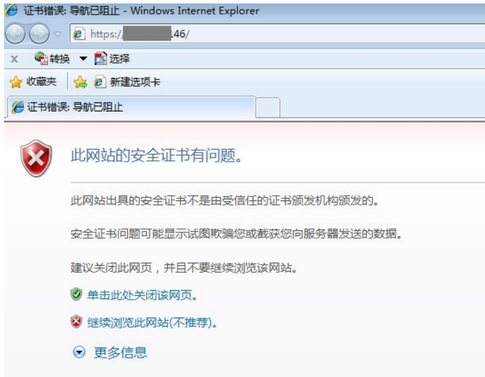
图3-36 证书错误
