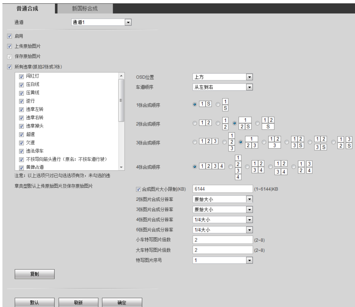
图3-10 普通合成
