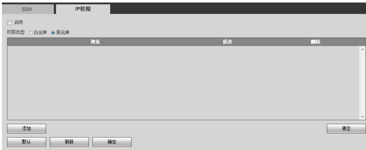
图3-64 IP 权限
