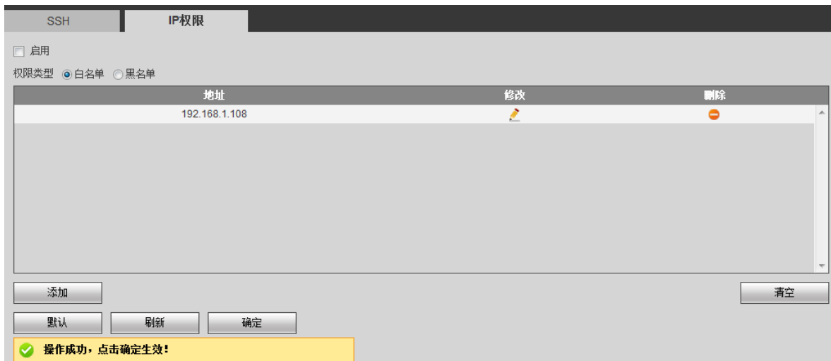
图3-66 白名单
