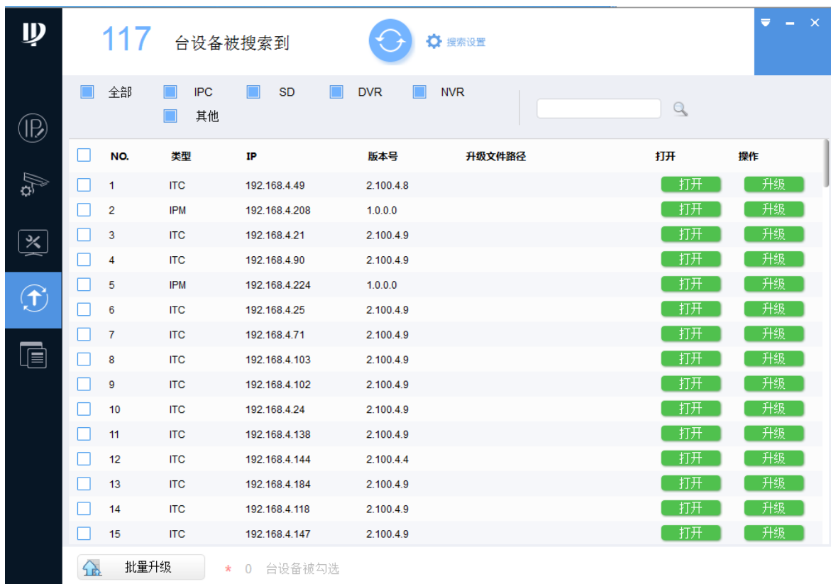
图2-9 升级
