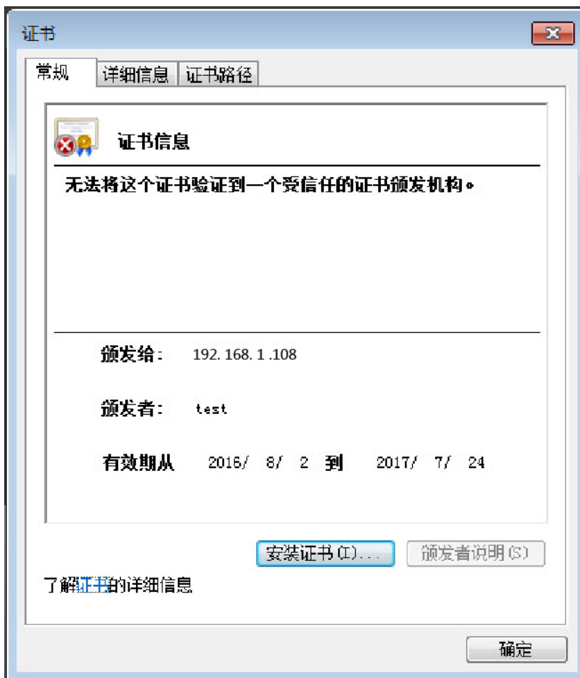
图3-28 证书信息
