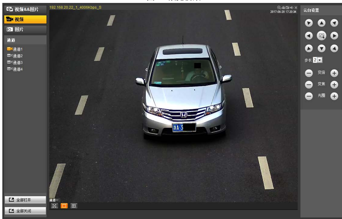
图3-3 预览视频
