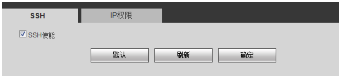
图3-63 SSH 界面
