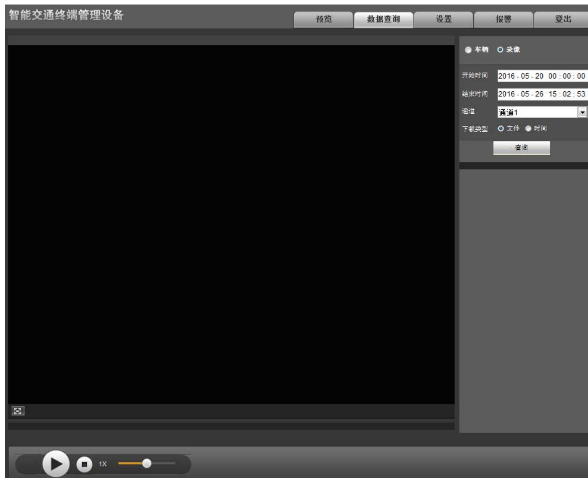
图3-8 查询录像
